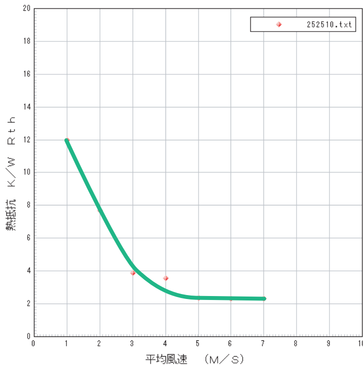
強制対流特性
