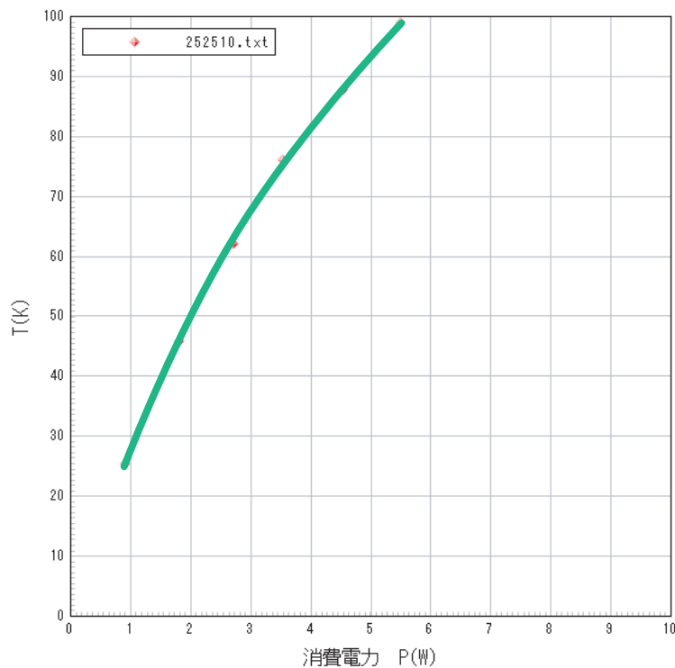
自然対流特性 室温 22℃
