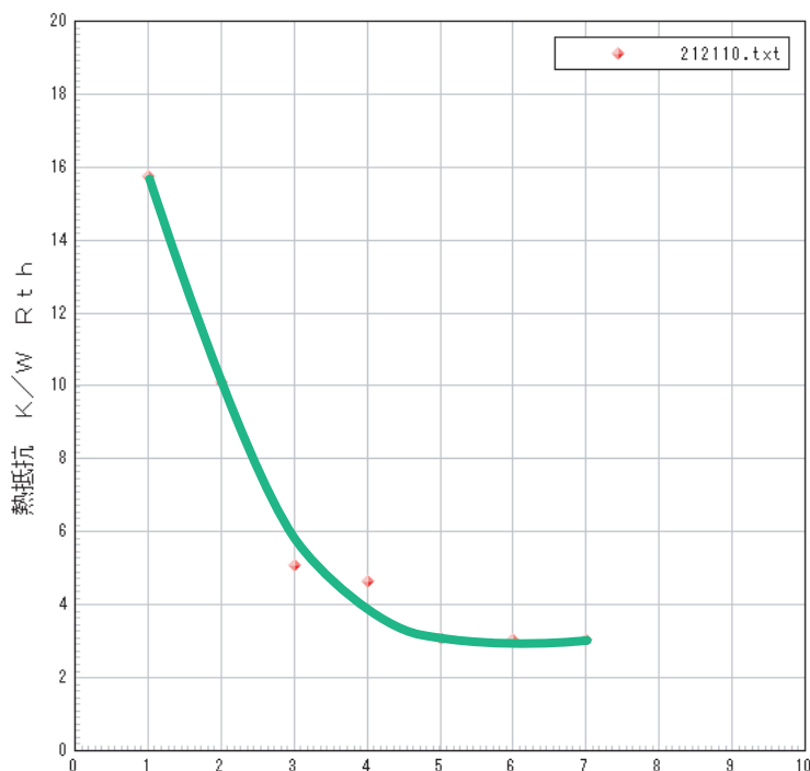
平均風速 (M/S) 強制対流特性
